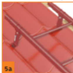
Установка кровельной лестницы на композитную кровлю
